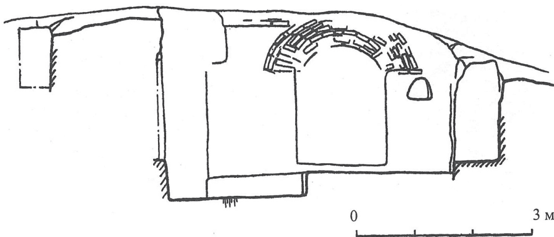
図 30. 部屋 22：断面図 11-11
