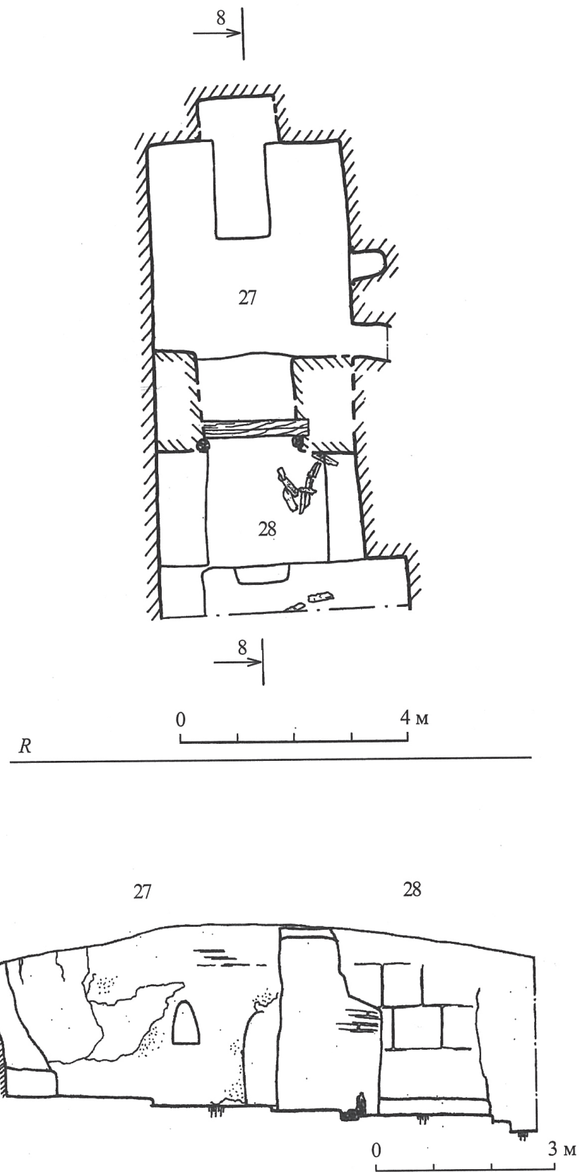
図 50. 複合体 D：平面プラン、断面図 8-8
