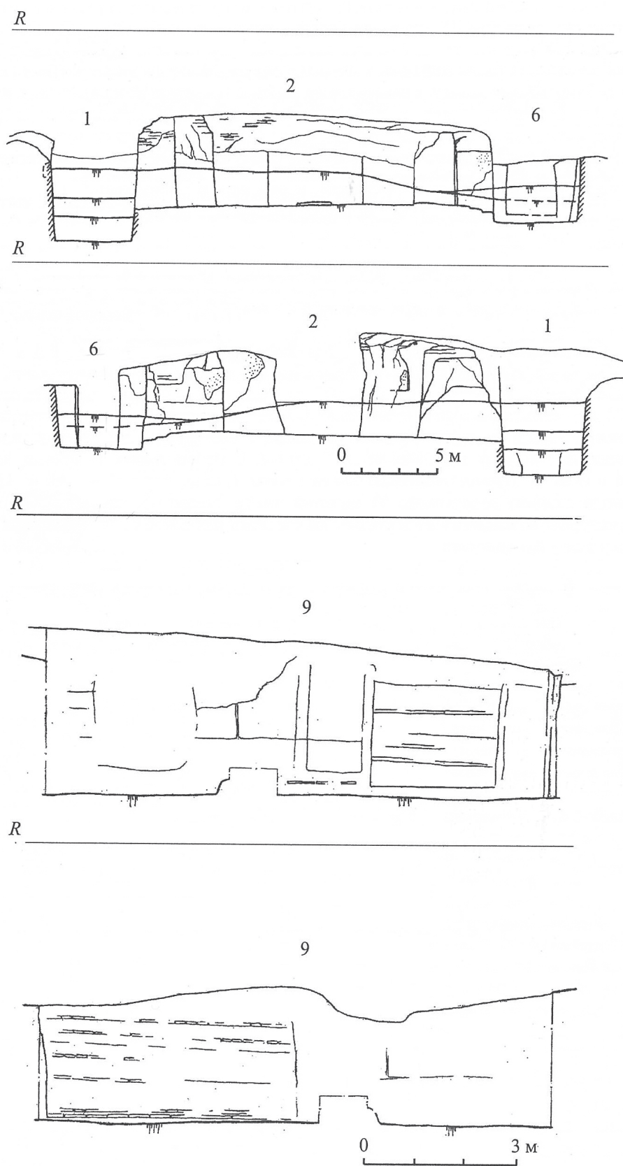
図 7. 断面図（部分）：3-3、3''-3''、4-4、4'-4'
