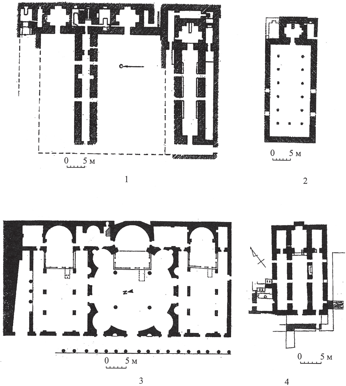
図 60. 教会の平面プラン
